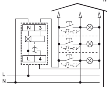
Collegamento a 3 fili
