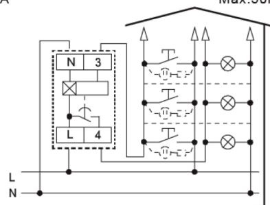
Collegamento a 4 fili
